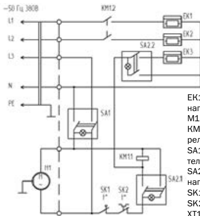
РИС. 5. СХЕМА ЭЛЕКТРИЧЕСКАЯ ZTV-9
