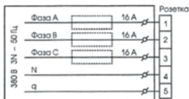
РИС. 8. СХЕМА ЭЛЕКТРИЧЕСКАЯ ZTV-15
